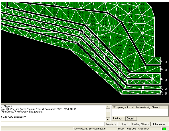
Complex Polygon Shape 에 대한 저항 계산 예시
