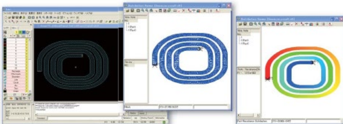
Spiral Polygon Shape 에 대한 저항 계산 및 Contour View 예시
